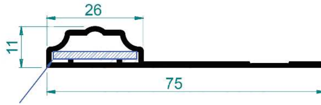
ÉQUERRE D'ASSEMBLAGE PIM001
